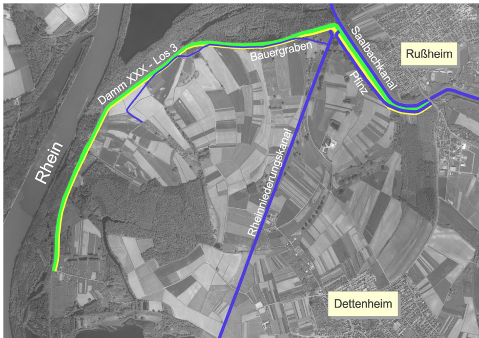
Übersicht Ausbau und Sanierung RHWD XXX, Los 3
