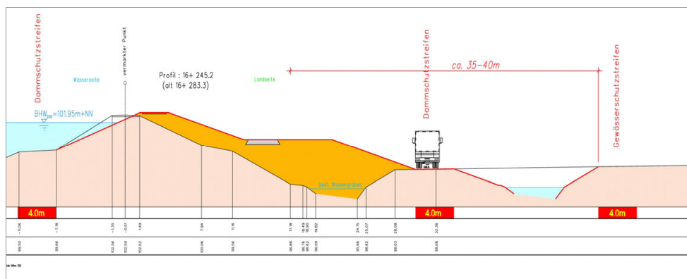
Regelprofil im Bereich der Pfinzverlegung
