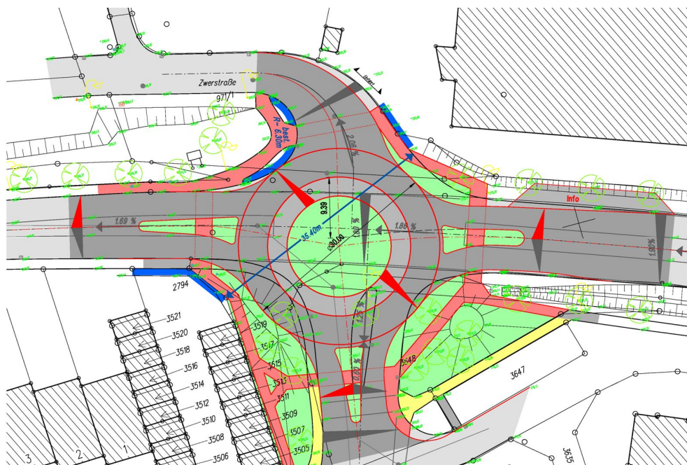
Lageplan Kreisverkehrsplatz
