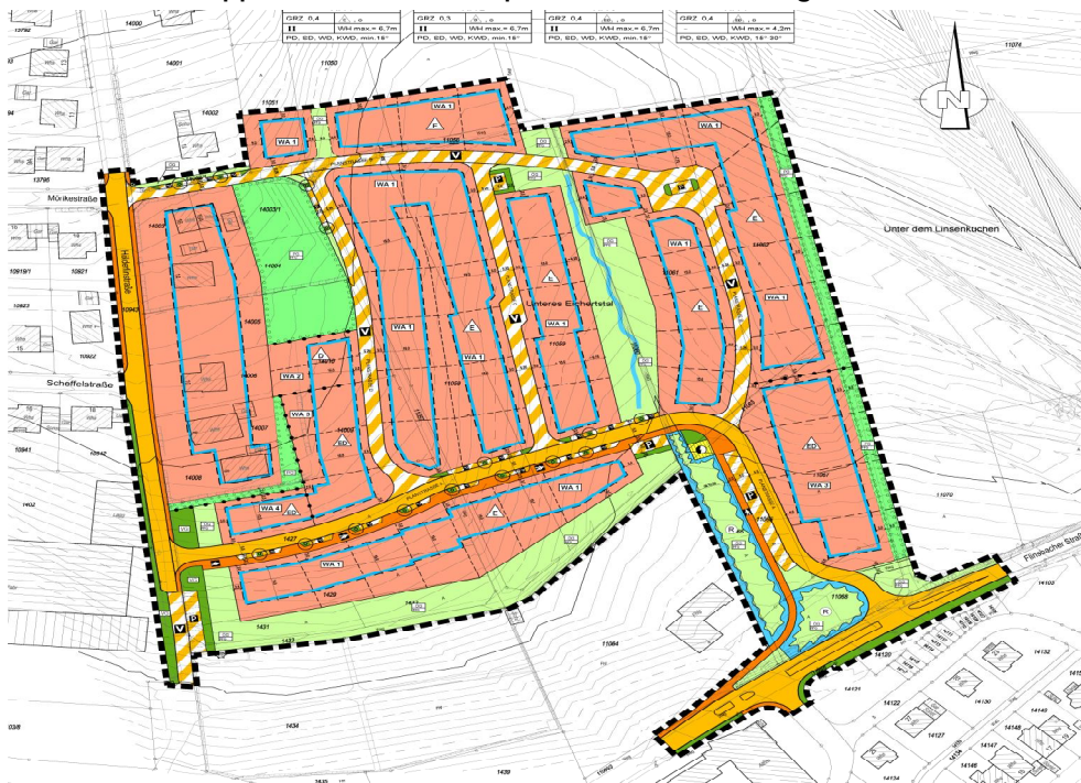
Bebauungsplan 07/2007
