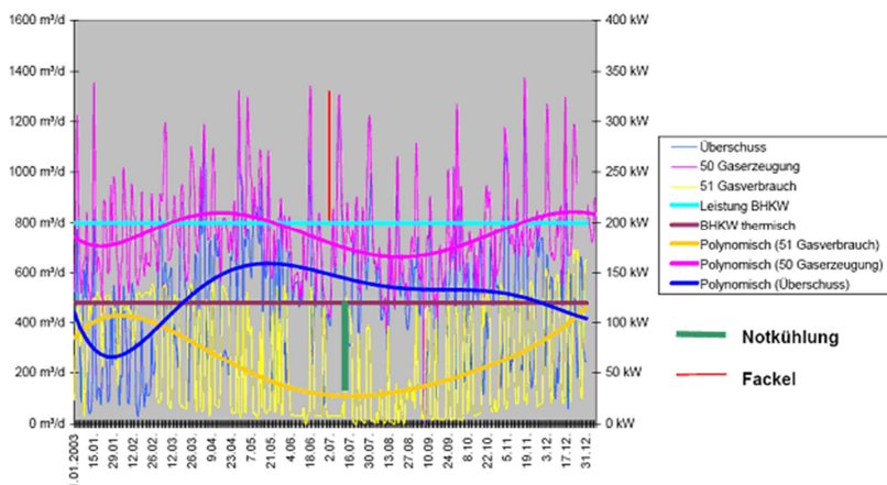
Klärgasanfall Waghäusel
